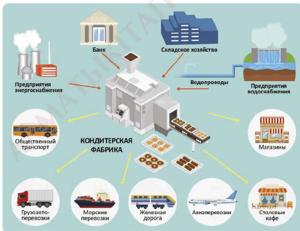
Рис. 61. Транспортная инфраструктура
